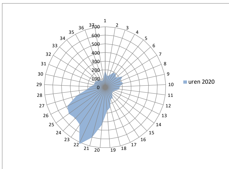
Figuur B3-1 Windroos op basis van metingen van het KNMI weerstation in Eelde, 2020.
